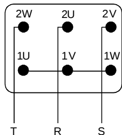
YY - 400V (P2)
