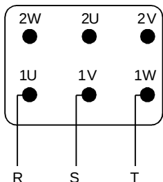
\Delta - 400V (P1)
